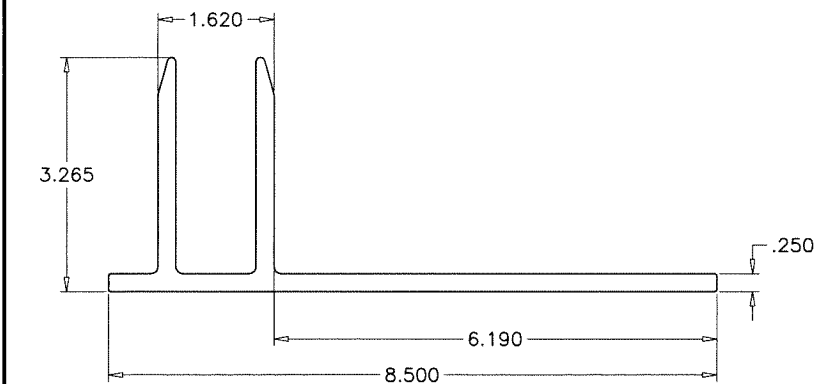
E28 JAMB ANCHOR
