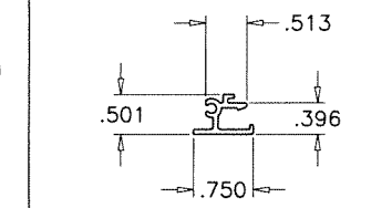
E19 VERTICAL SPACER
