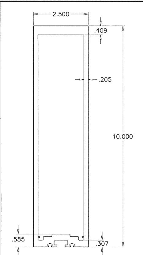
E17 JAMB/MULLION
