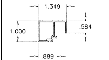
E22 GUIDE
