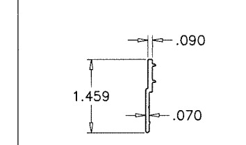
E19 VERTICAL SPACER
