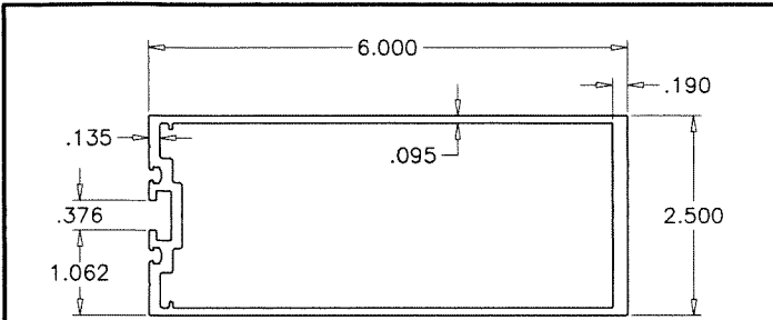
E16 HEAD/SILL/HORIZONTAL
