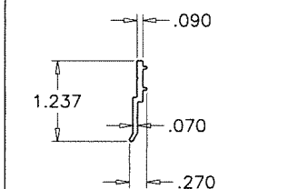
E32 FLANGE TOP
